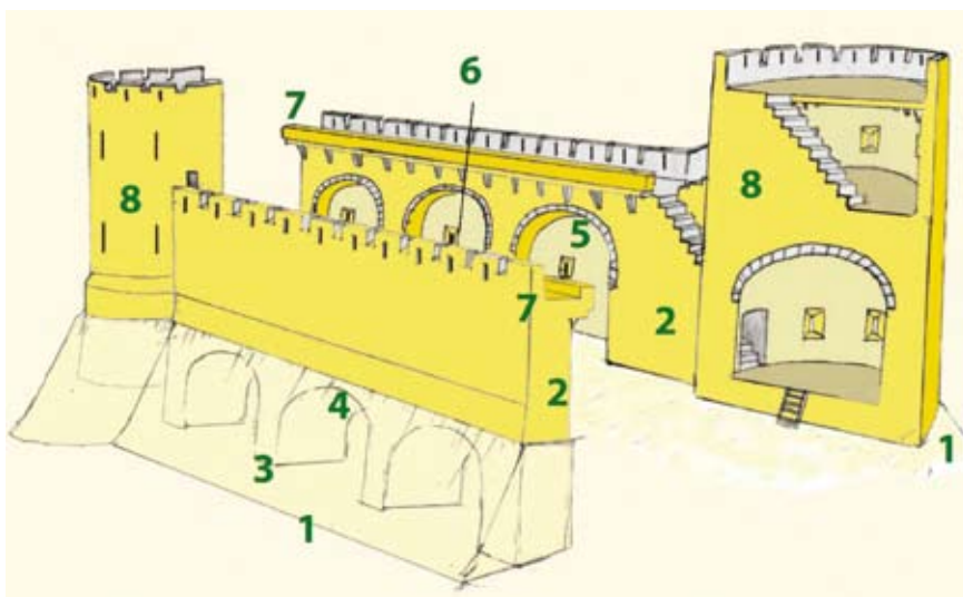
Onderdelen van een middeleeuwse stadsomwalling : 1. walgracht, 2. walmuur, 3. funderingspijler, 4. funderingsboog, 5. steunboog, 6. schietgat, 7. weergang, 8. toren (uit: Wandelen langs de eerste omwalling, Brussel Stedelijke Ontwikkeling)
