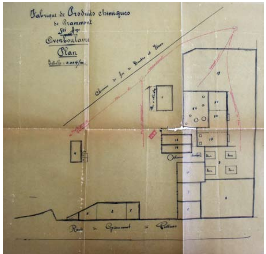
Gedetailleerd grondplan van de ‘Zwartfabriek’, opgemaakt door landmeter Omer De Boe op 19 februari 1921
