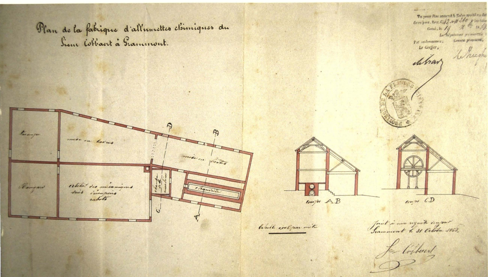
Grondplan van het lucifersbedrijf van François Cobbaert, ingediend bij zijn aanvraag bij het provinciebestuur voor het plaatsen van een zwaardere stoommachine en dito ketel. De werkruimte voor het inpakken van lucifers in dozen (CD) ligt een niveau lager dan het stoomhuis met machine (AB) (31 oktober 1868).
