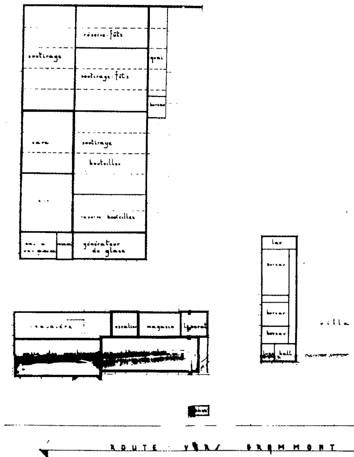
Afb. 7: grondplan van Brouwerij "Dendria", dd. 17 juli 1940: niet op het plan: "cheminée", uiterst links tussen beide hoofdgebouwen; onleesbaar in het voorgebouw v.l.n.r.: "salle des machines (à vapeur)", "salle de brassage", klein gebouwtje helemaal vooraan: "essence"
